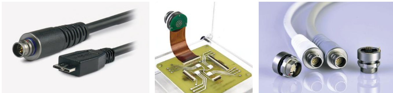
Рис.7. Примеры сборок ODU AMC High-Density. Патч-корд с разъемом RJ45 – а; монтаж розетки на гибкий шлейф – б; монтаж с кабелями разного цвета – в
